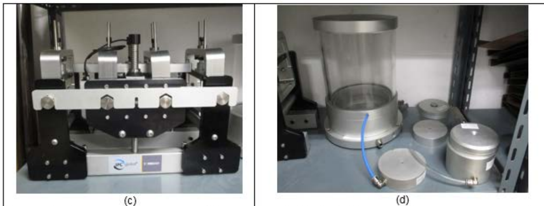
Figura 2. Utensilios de ensayos adquiridos con la máquina AMPT para la realización de los diferentes ensayos.
