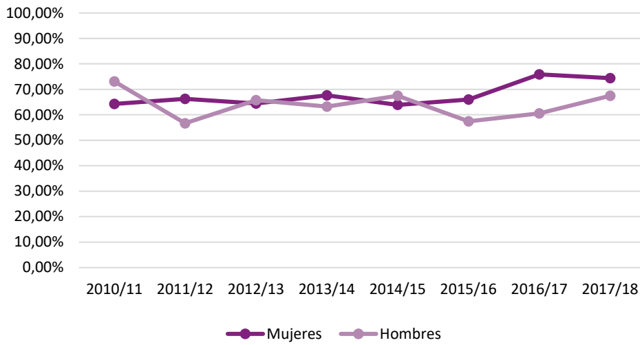
Gráfico 239. Evolución de la tasa de rendimiento del Grado en Ingeniería de los Recursos Mineros por sexo, 2010/2011-2017/2018
